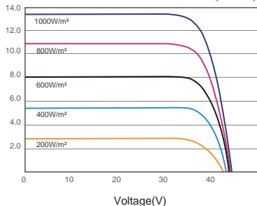
I-V CURVES OF PV MODULE(480W)
